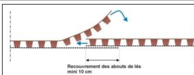
Figure 12 - Recouvrements transversaux (abouts de lés)
