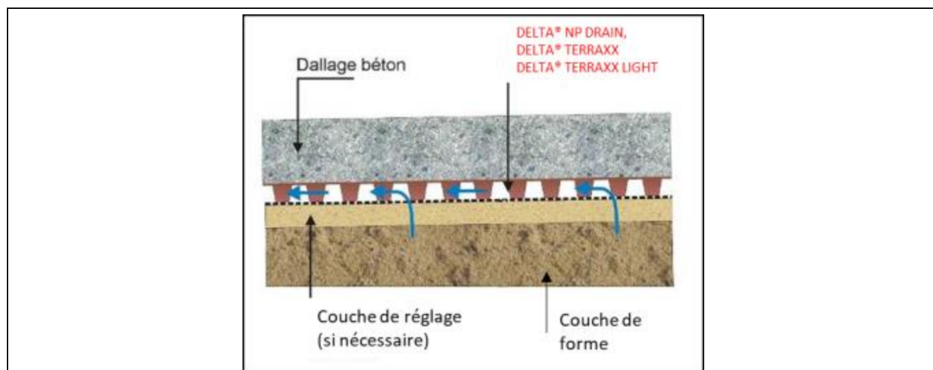
Figure 3 – Principe de mise en œuvre sous dallage béton
