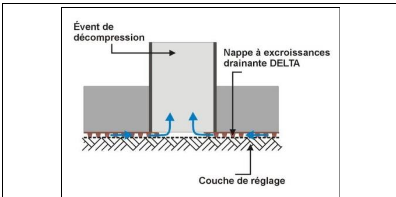
Figure 17 - Event de décompression
