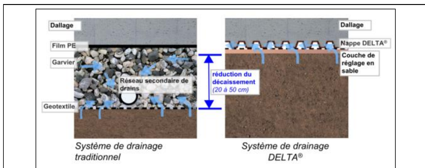
Figure 5 - Comparaison du système traditionnel dits des « hérissons drainants » et du système DELTA®
