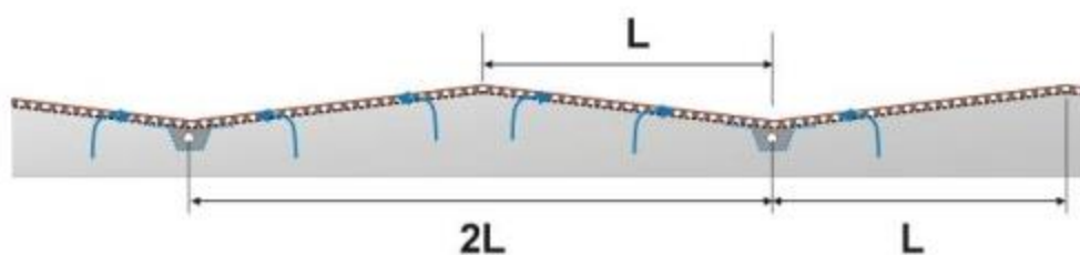
Figure 6 - Visualisation de la distance maximale d'écoulement
