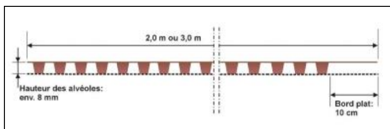
Figure 8 - Vue en coupe de la nappe DELTA®-NP DRAIN
