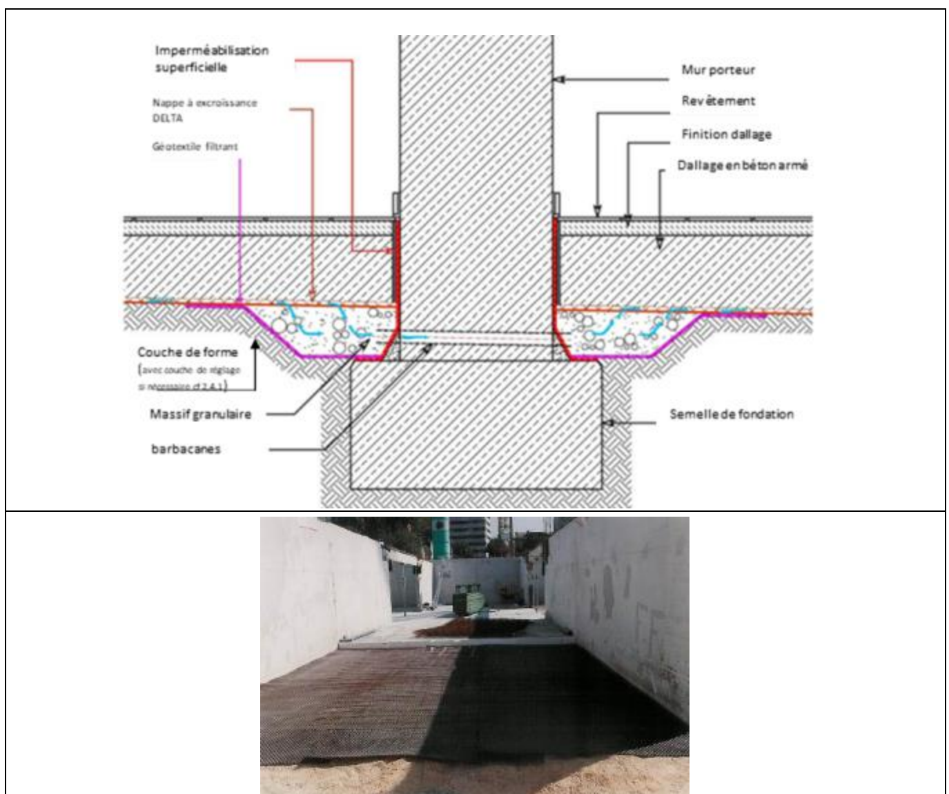
Figure 14 - Raccord au niveau de murs de refend / dallage désolidarisé
