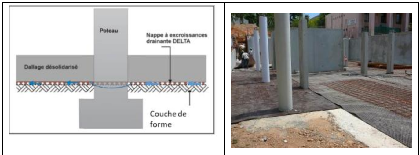
Figure 13 - Raccord au niveau de poteaux
