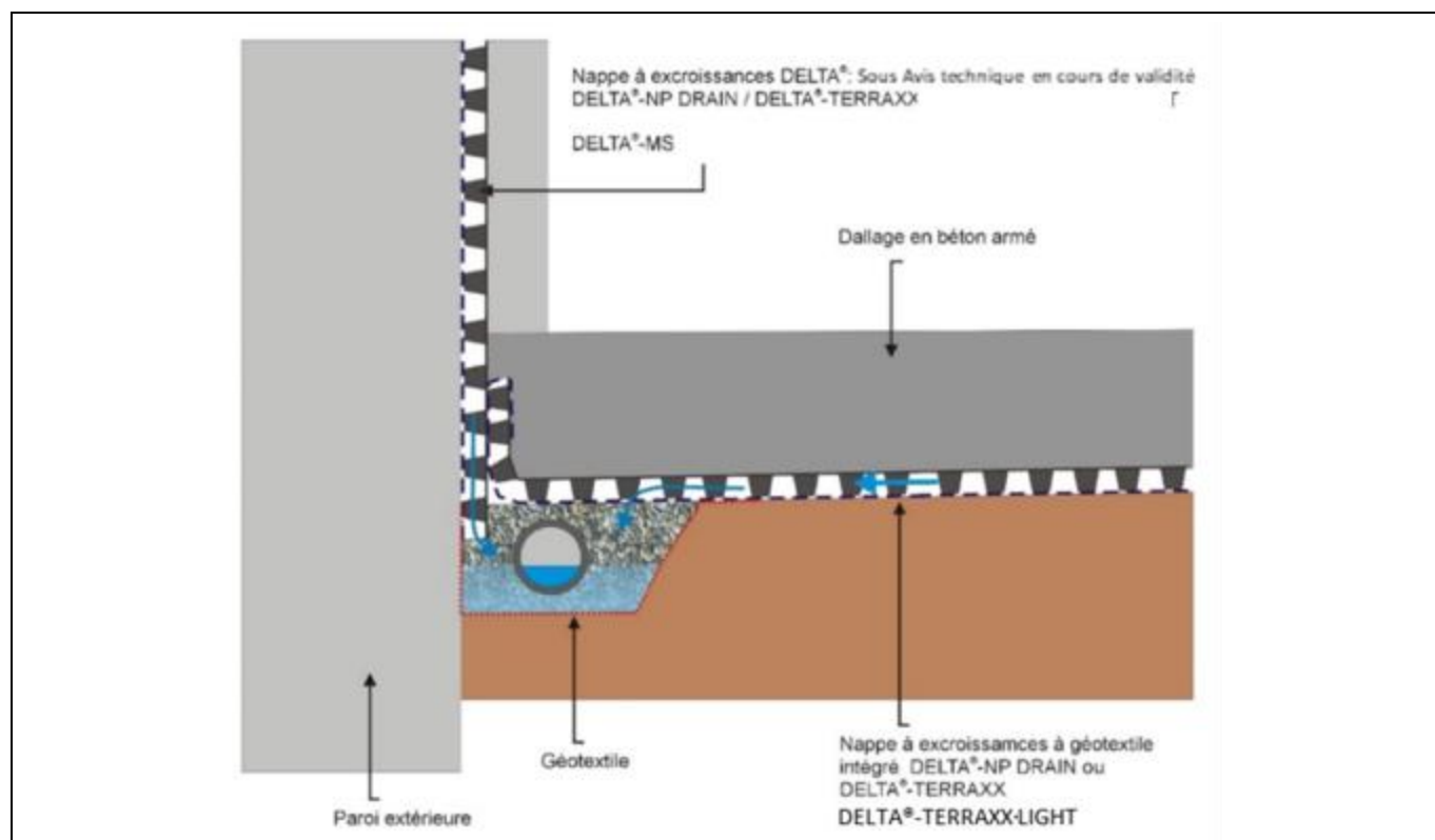
Figure 15 - raccord du dallage à une paroi extérieure
