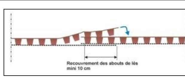
Figure 12 - Recouvrements transversaux (abouts de lés)
