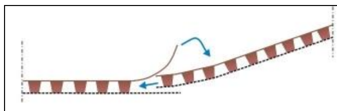
Figure 9 - Vue en coupe de la nappe DELTA®-TERRAXX et DELTA®-TERRAXX LIGHT
