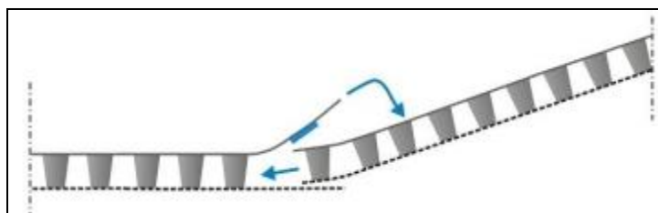
Figure 10 - Recouvrements longitudinaux de la nappe DELTA®-NP DRAIN
