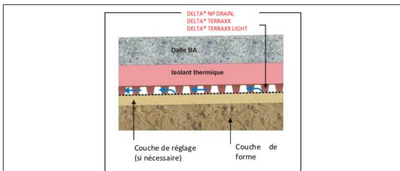
Figure 4 – Principe de mise en œuvre sous dalle béton sur isolant
