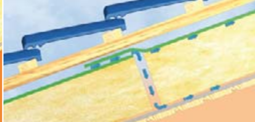
Ohne Verklebung dringt Kälte ins Dach.
